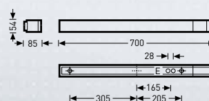
Acuro St(-S) 114...01
