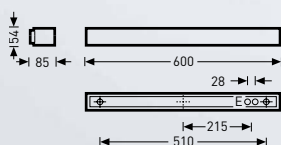
Acuro 114...
