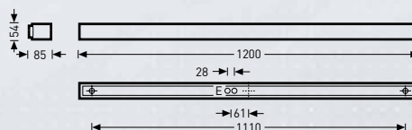
Acuro 139...
