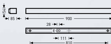
Acuro 128...
