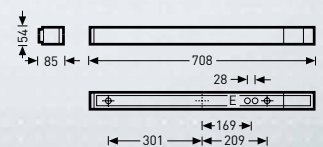
Acuro St(-S) 114...04
